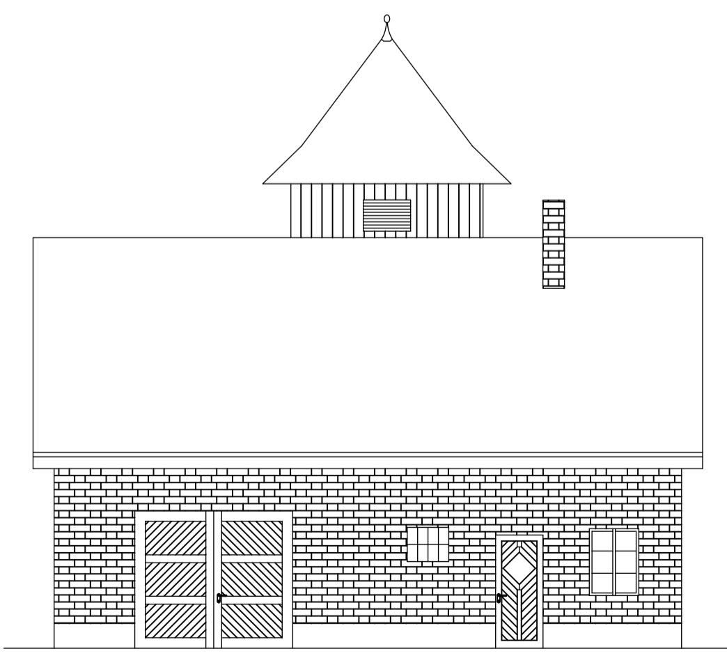
Ost - Ansicht
