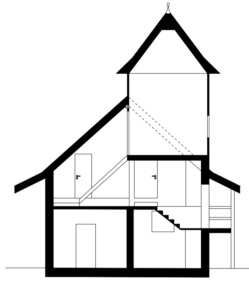
Schnitt B
