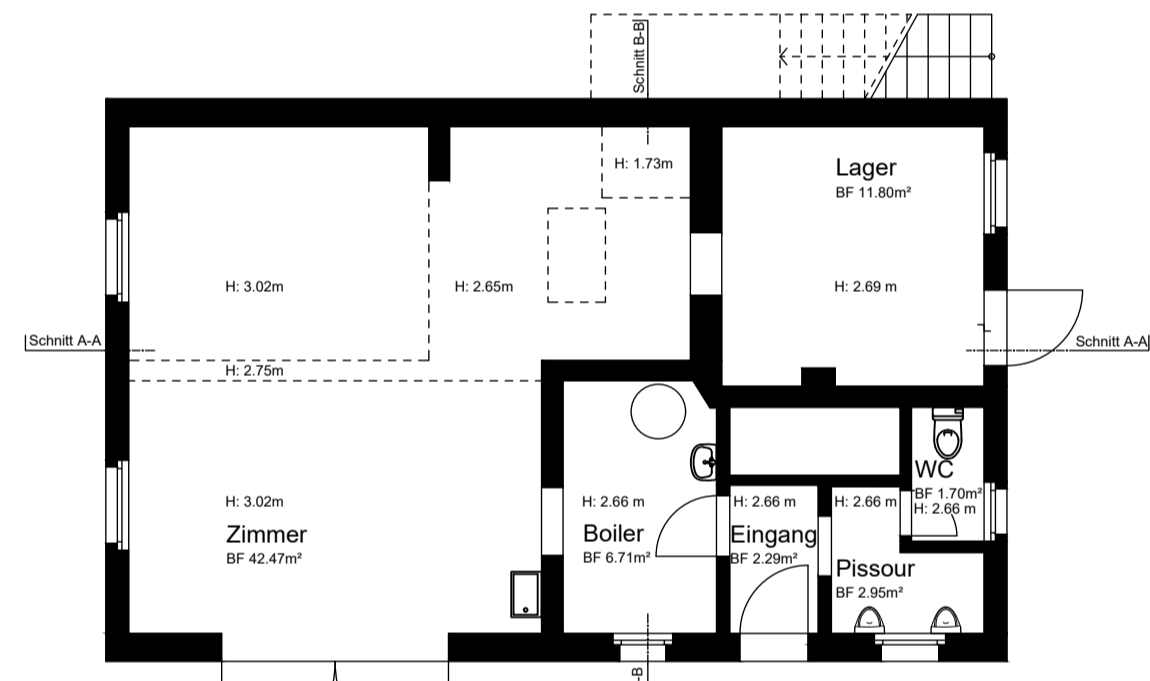
Erdgeschoss
