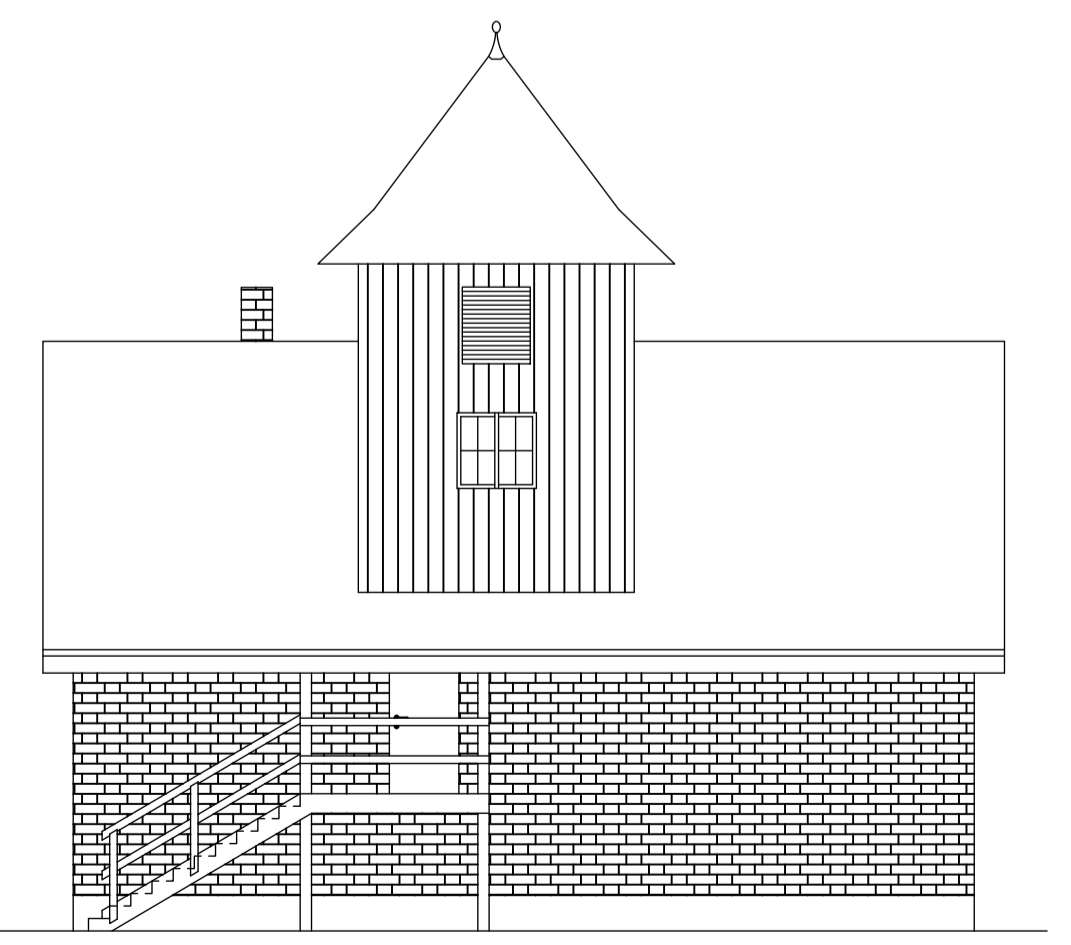
West - Ansicht
