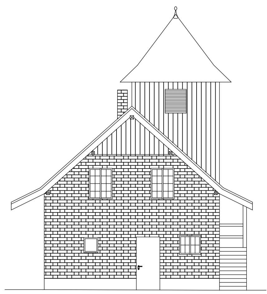
Nord - Ansicht
