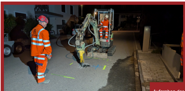
Aufgraben der beschädigten Leitung
